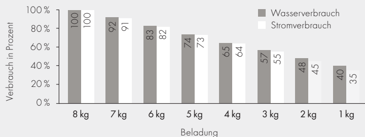
Einsparung durch Teilbeladungs-Sparautomatik
